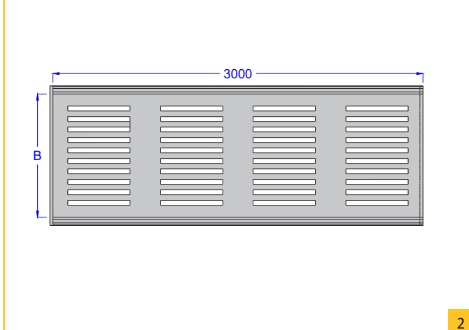
BOVENAANZICHT BODEMPLAAT
